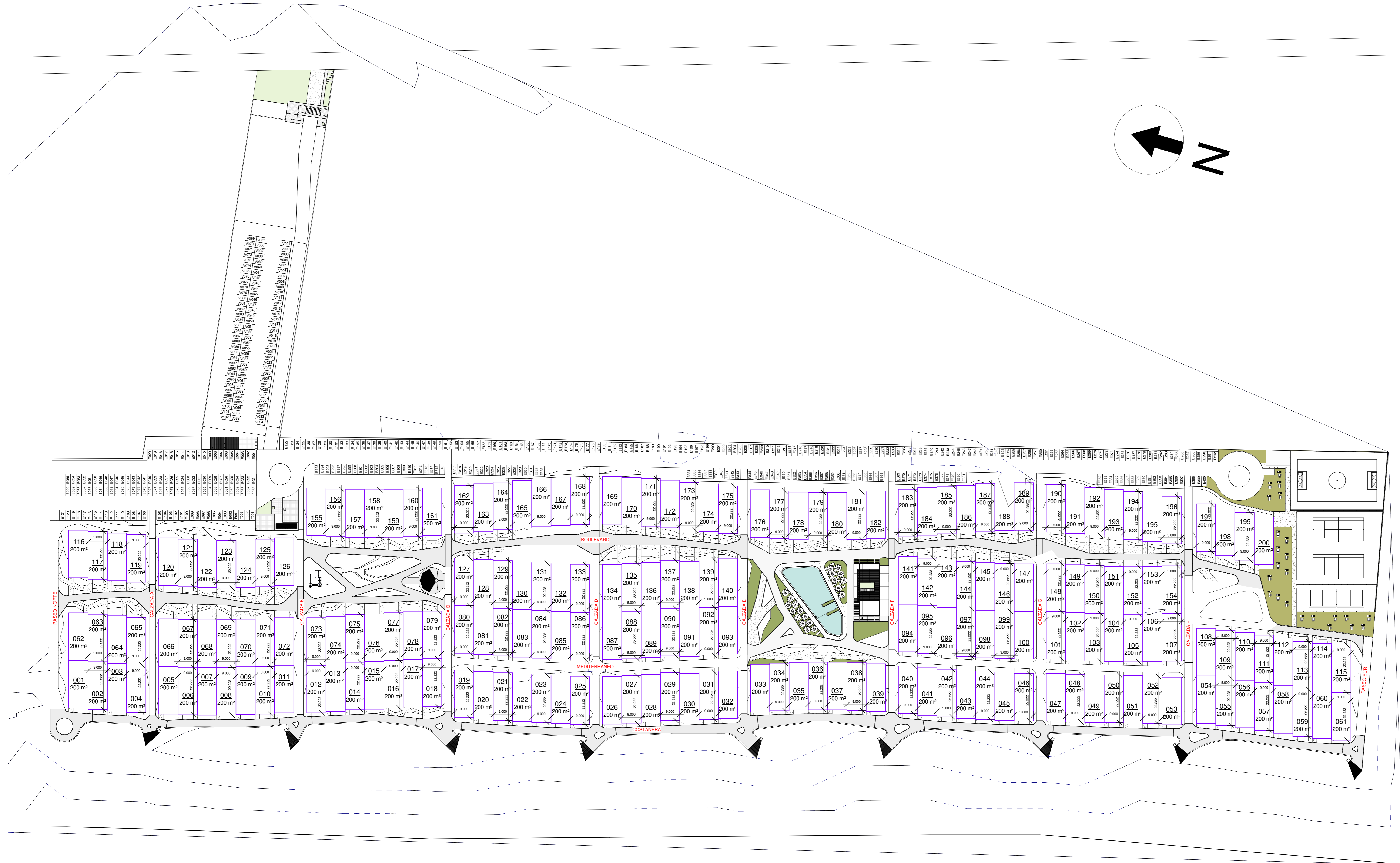
1 PLANO DE LOTIZACIÓN MP-M03 1: 750
