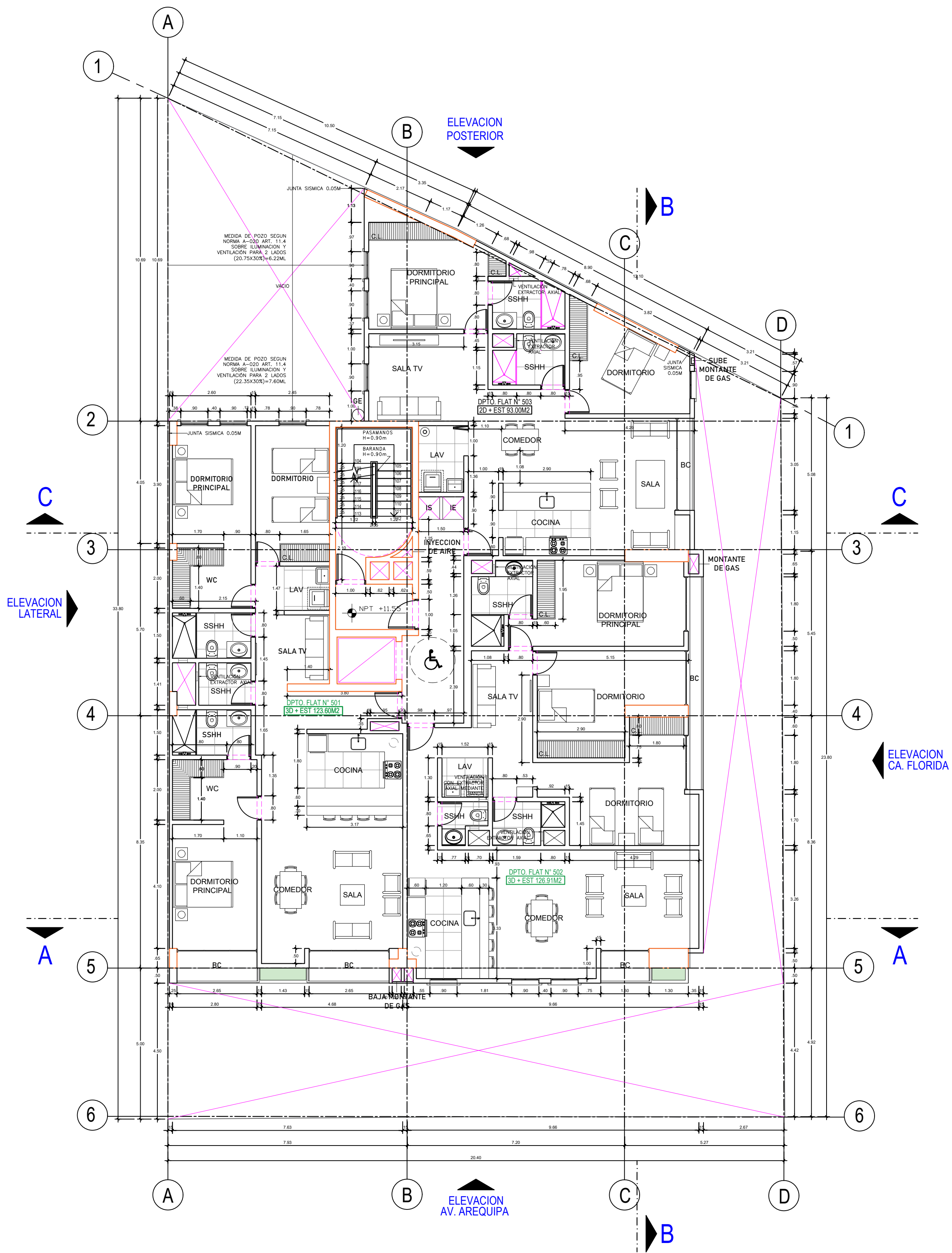
PLANTA 5
