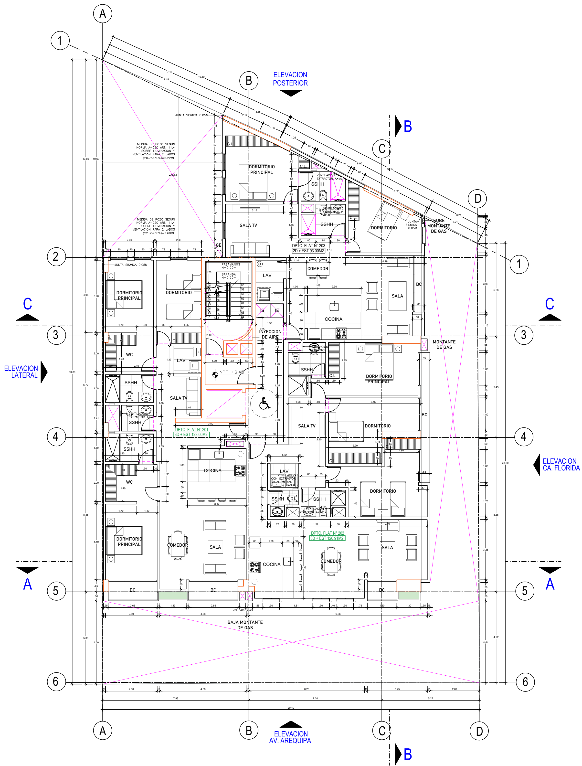
PLANTA 2
