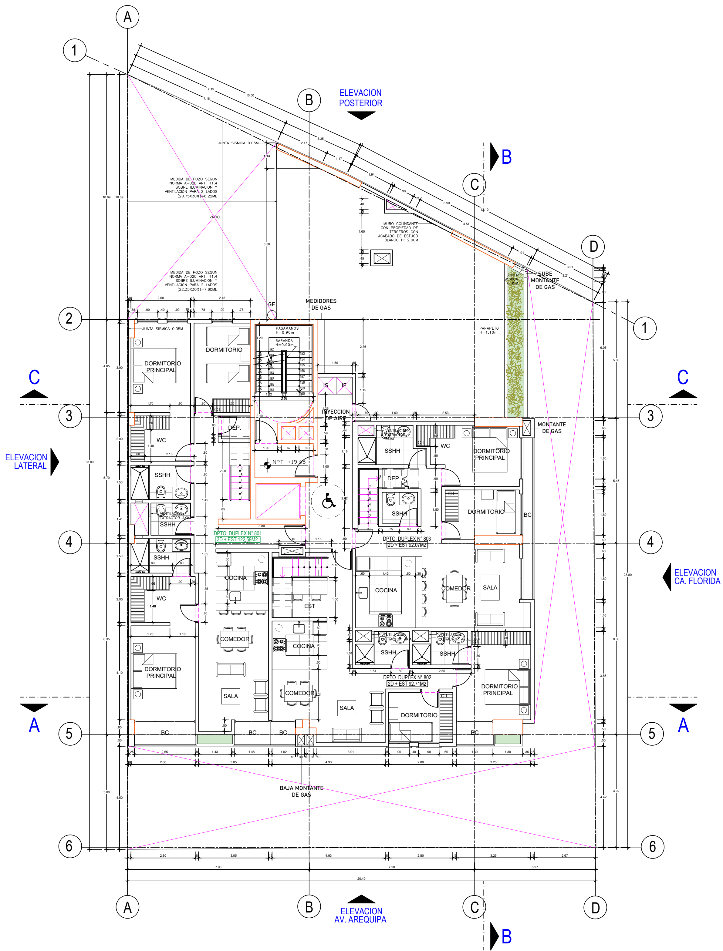
PLANTA 8
