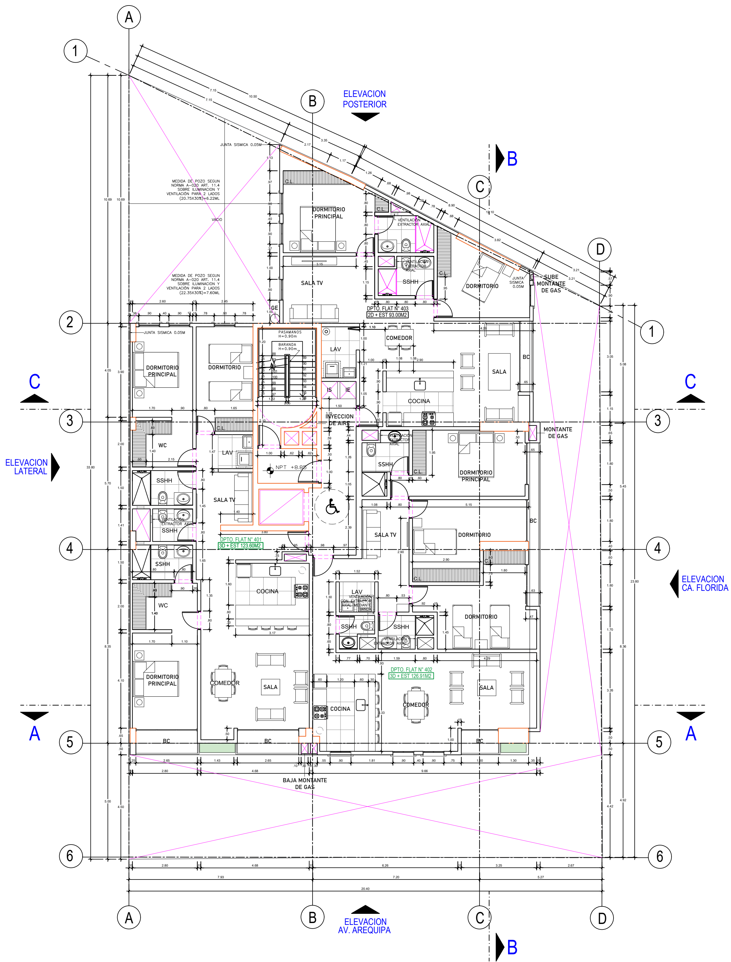
PLANTA 4
