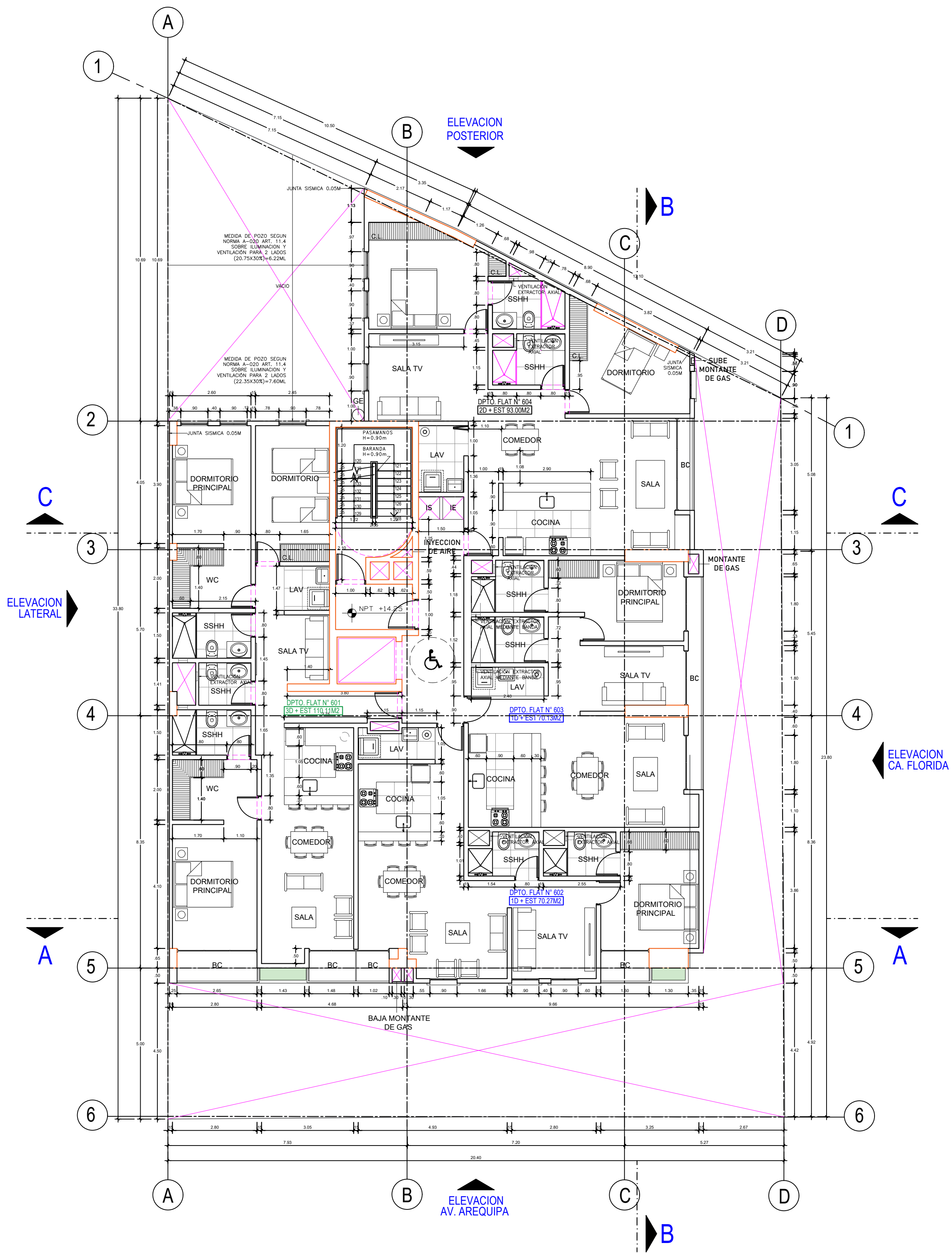
PLANTA 6
