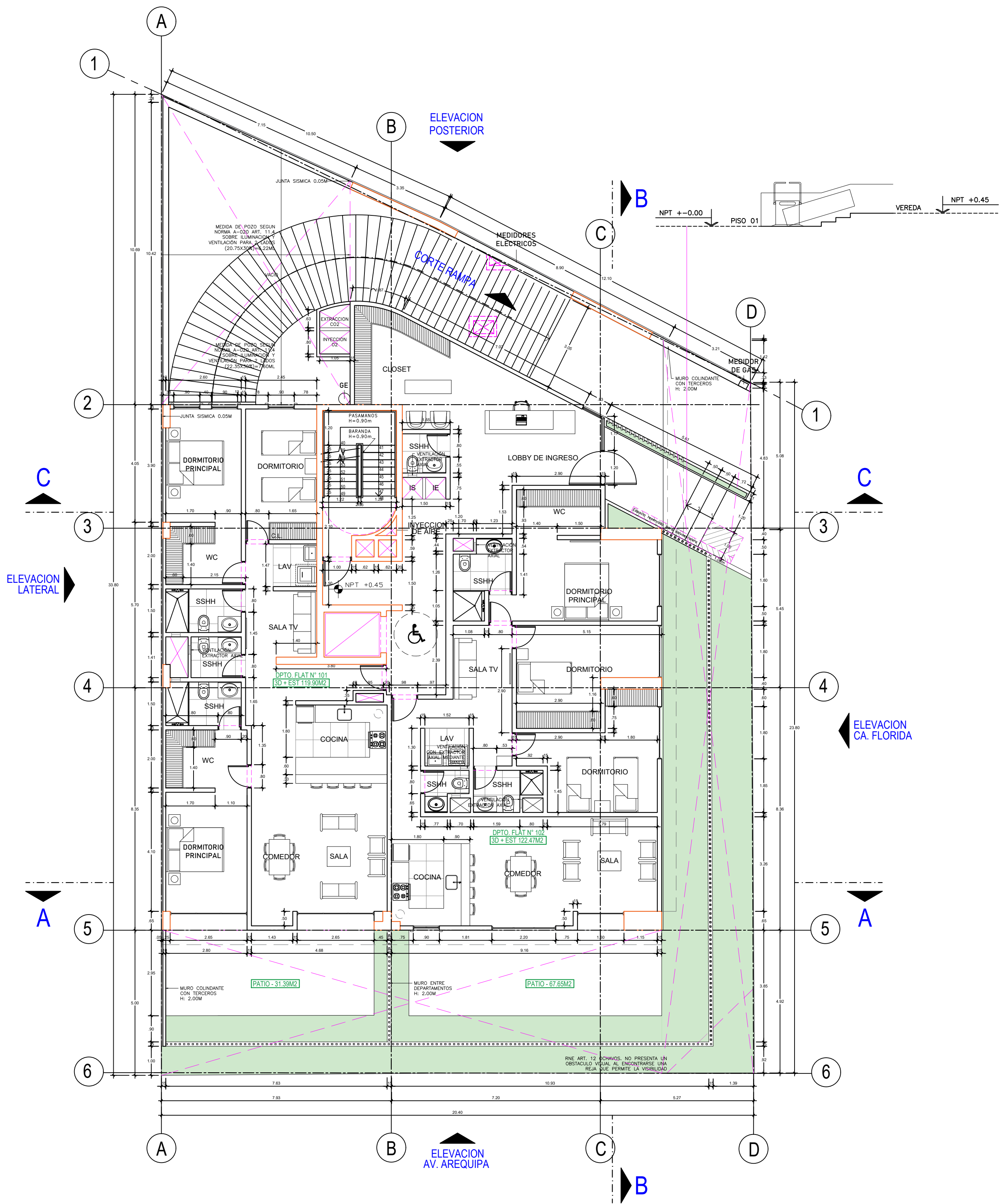
PLANTA 1
