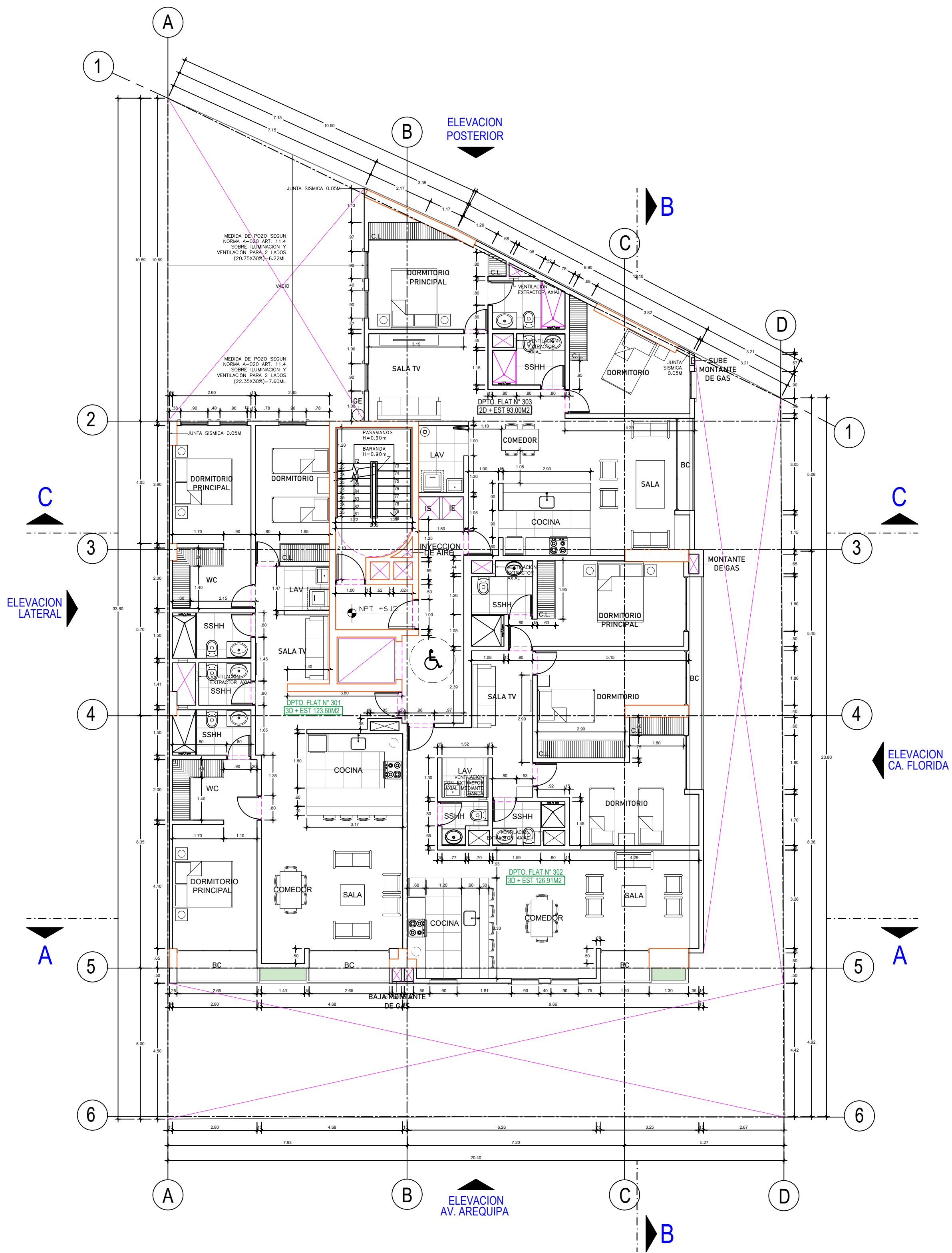
PLANTA 3
